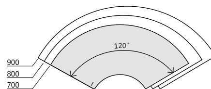
120° with intercut | 120° z wcięciem
